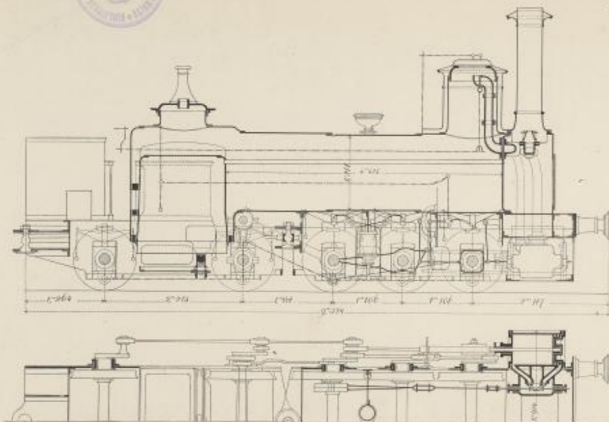
Type 34. gebaut 1862. SEYDLER & ENGELHARDT
