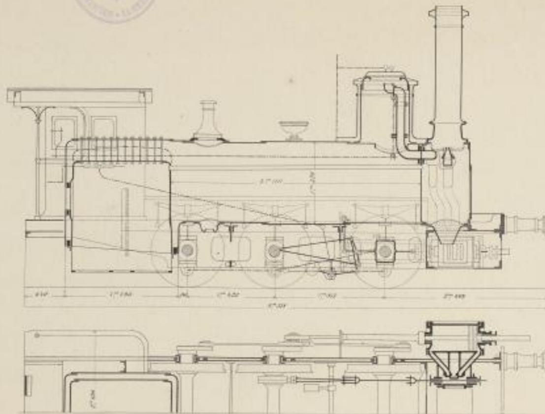
Type 42. gebaut 1868. Fabrik in Maschinen-Fabrik.
