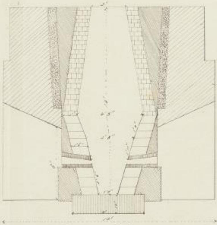
Längen - Durchschnitt
