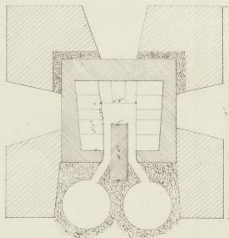
Horizontal - Durchschnitt
