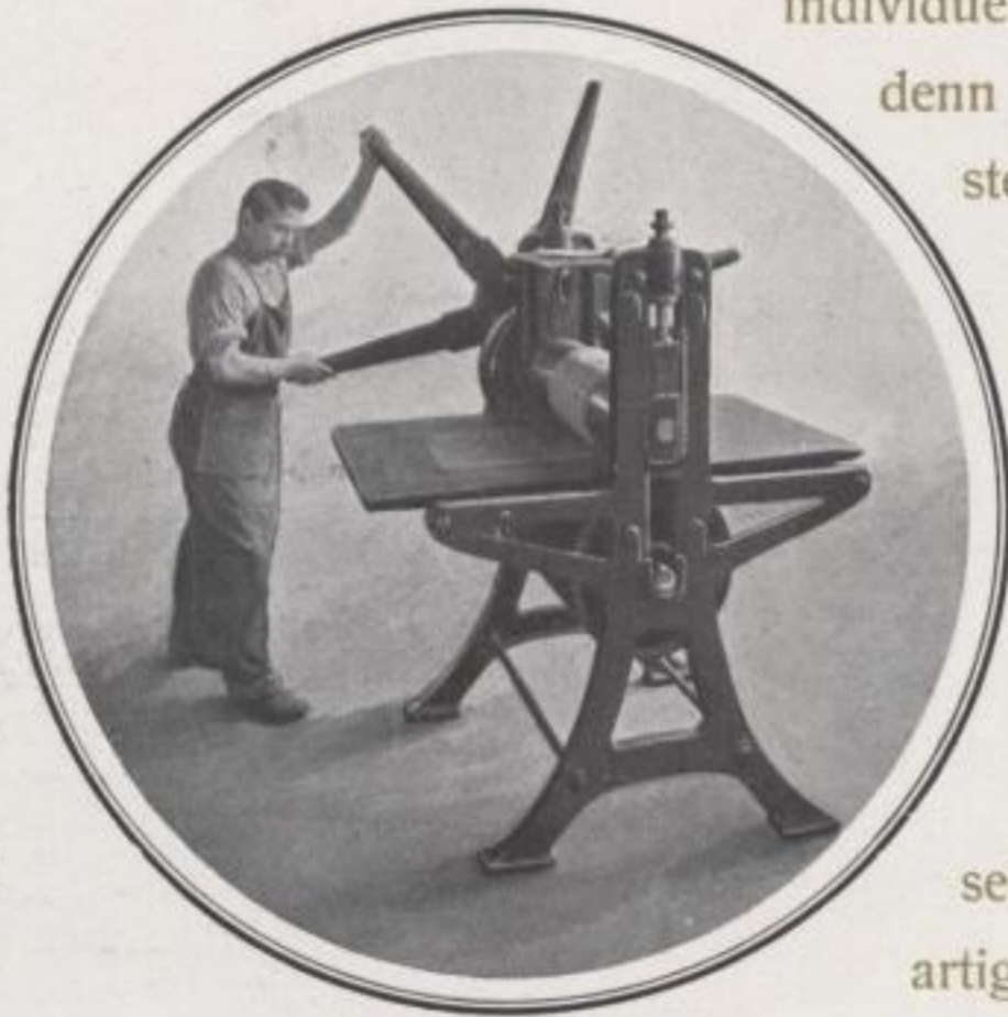
Sterndruckpresse für Kupferdruck.
