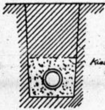
Dränleitung
