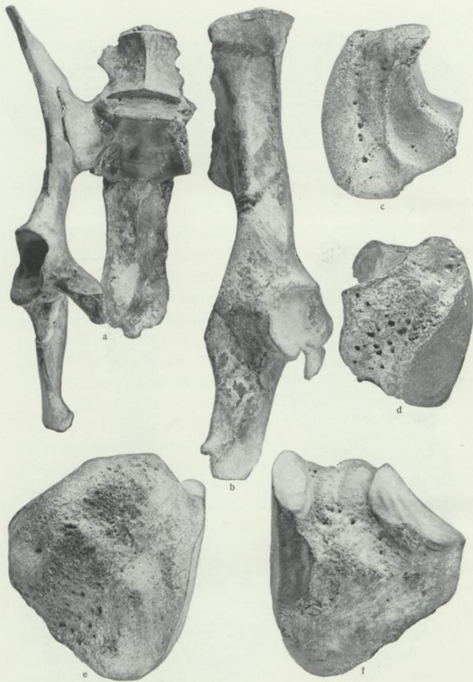
Abb. 119. Pleistozäne Fossilien aus der Quebrada de Chalang bei Punin: a) und b) Rechte Beckenhälfte mit letztem Lendenwirbel und Kreuzbein von Cervus sp.; \frac{1}{2} n. Gr., c) und d) Carpalknochen von Mylodon sp.; \frac{5}{9} n. Gr., e) und f) Scaphoid von Mastodon sp.; \frac{1}{2} n. Gr. Aus der Sammlung von Hans Meyer im Paläontologischen Institut der Universität Leipzig.
