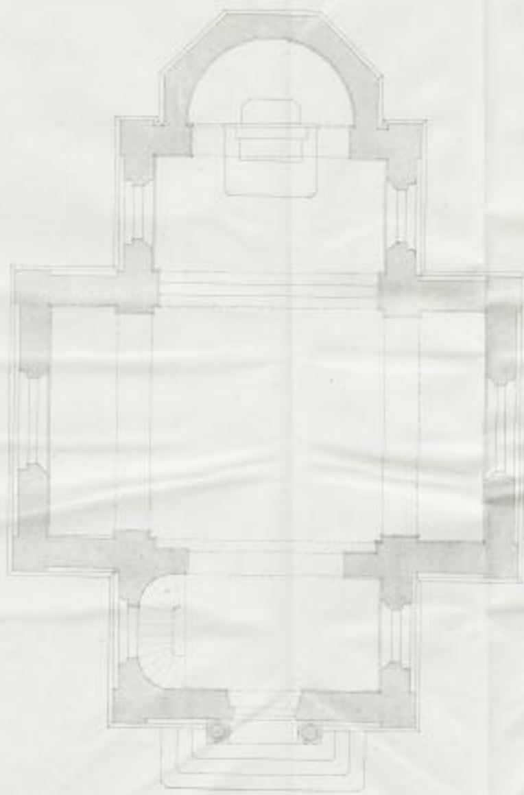
Grundriss Parterre.
