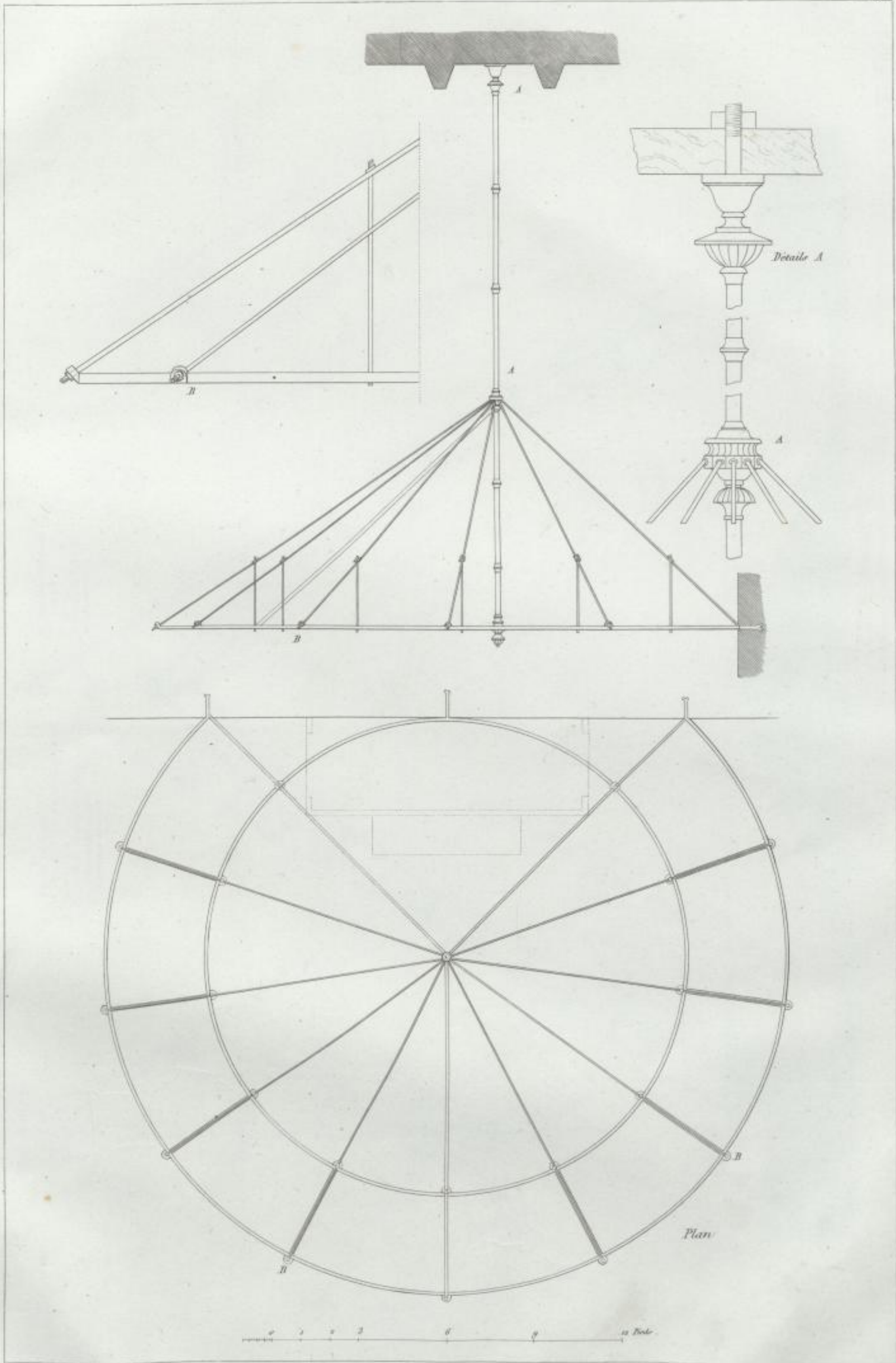
Armature en Fer supportant les Lampes dans les salles des Concours de l'Ecole du Palais des Beaux-Arts.
