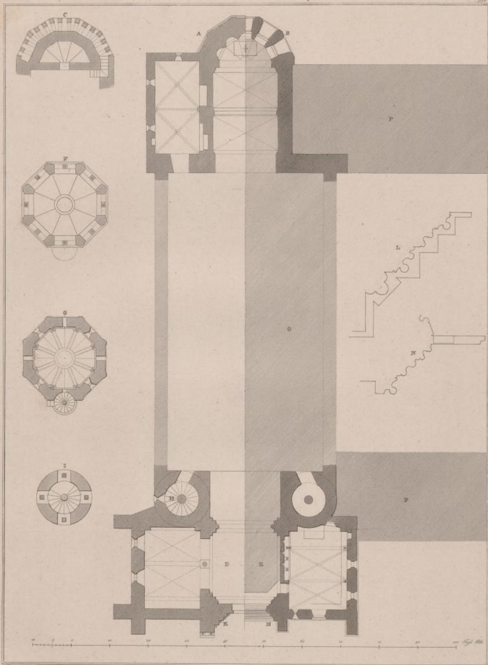
Grundriß der St. Paulskirche zu Worms
