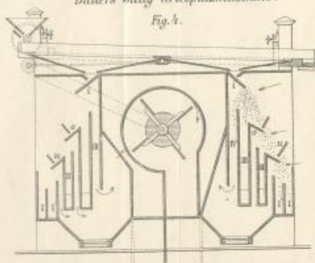
Bauers Saug-Griesputzmaschine.
