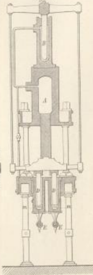
Hydraulische Maccaroni Presse Fig. 7 a.
