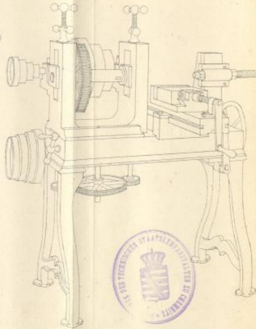
Fraismaschine.
