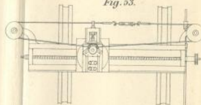
Sharp Stewart & Co. Support Detail zur Hobelmaschine nach Sellers' System.
