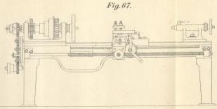
H. Hind & Son. Supportdrehbank.
