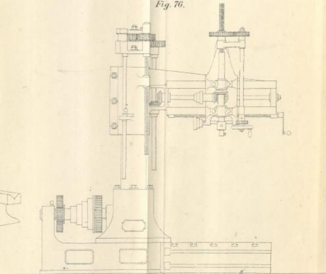
D. New & Co. Radialbohrmaschine.
