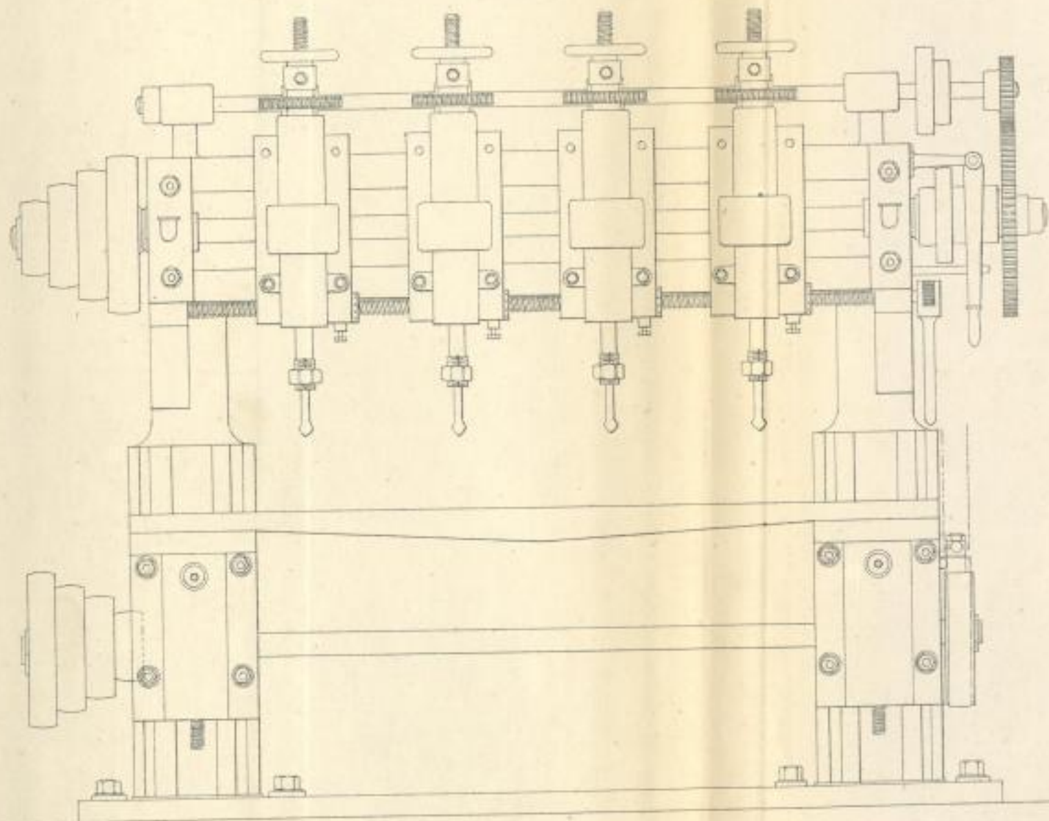
Verticalbohrmaschine mit vier Spindeln von Bede & Co.
