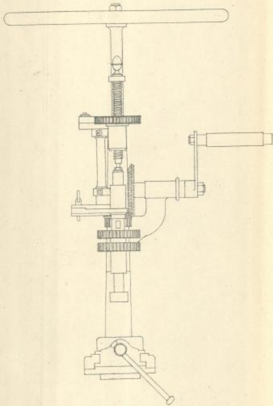
Bohrmaschine von Daudoy, Mailliard, Lucq & Co.
