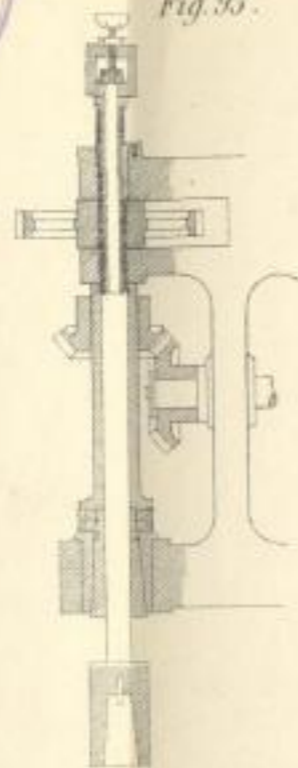
Bohrspindel
