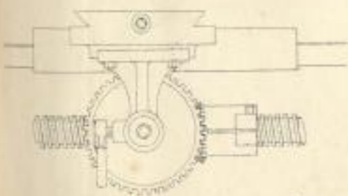
Schloss
