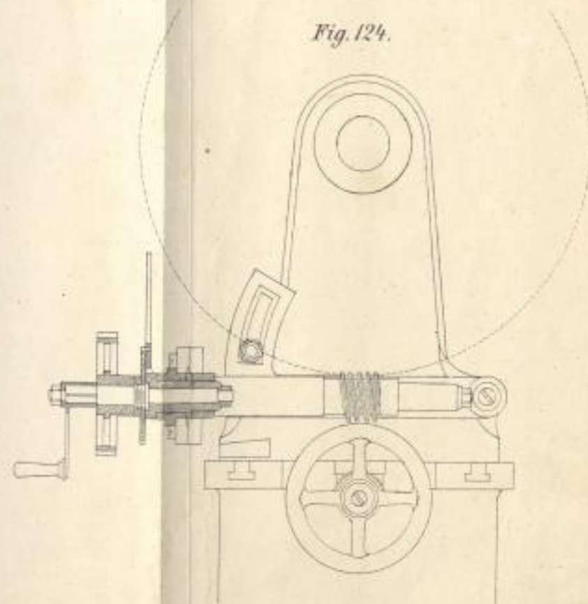
Schrägträderhobelmaschine von Leupold.
