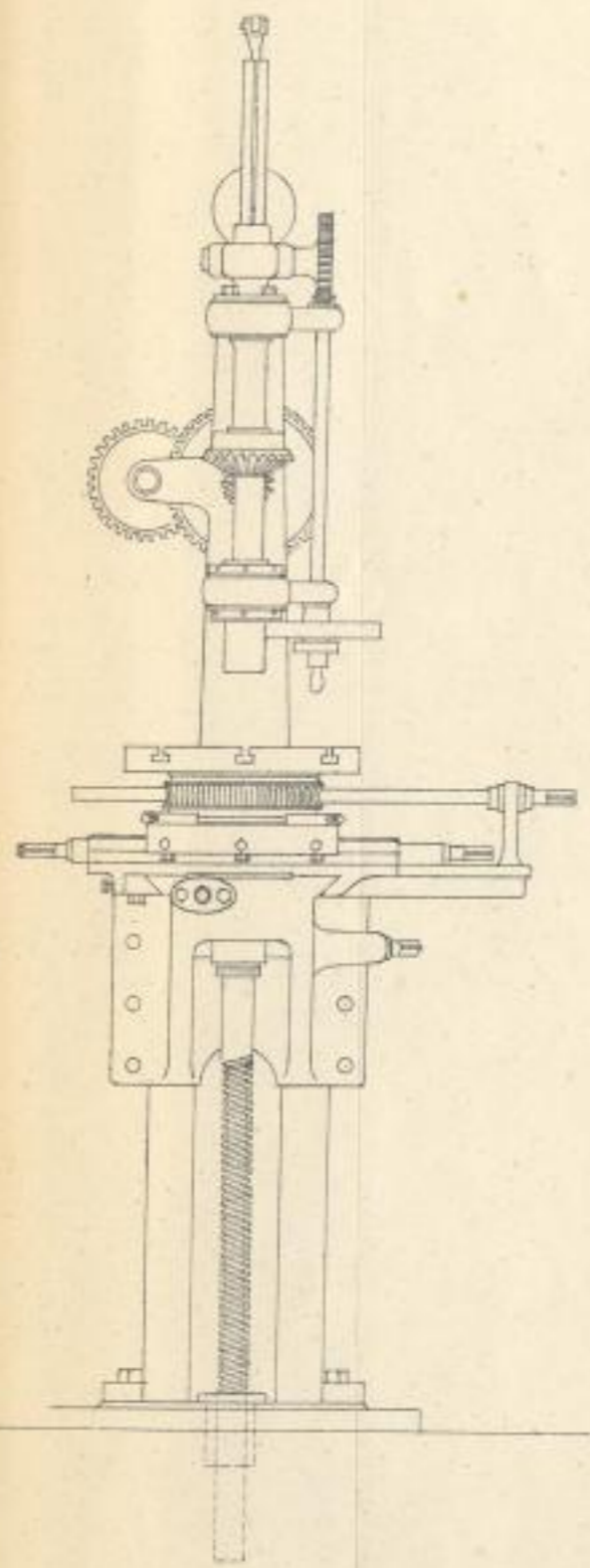
Freistehende Bohrmaschine von Heilmann-Ducommun & Steinleu
