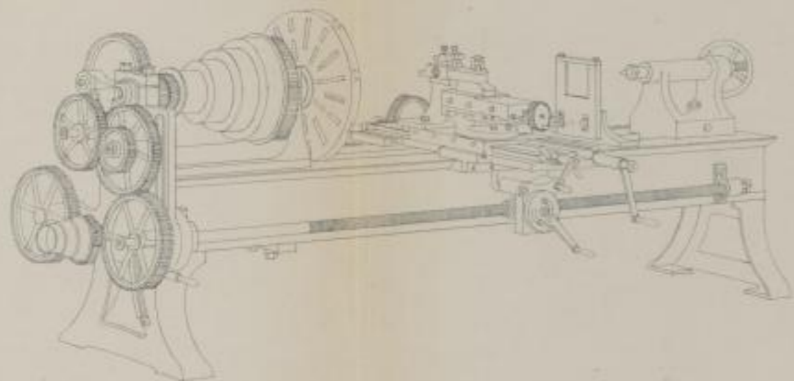
Suportdrehbank und kleine Shapingmaschine von Gschwindt & Co.
