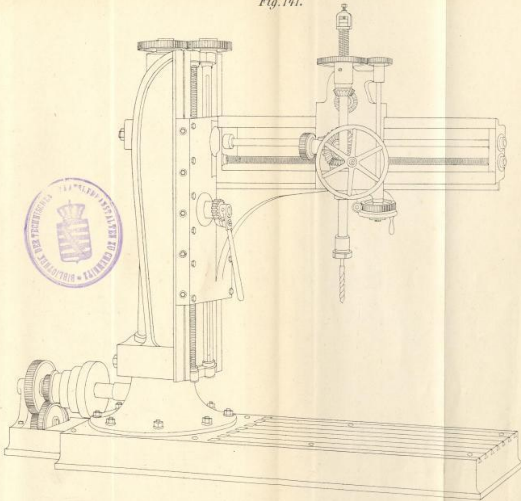
Grosse Radialbohrmaschine von Gschwindt & Co.
