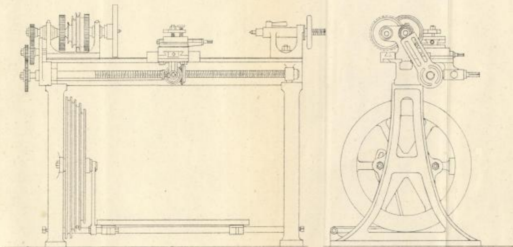
Fussdrehbank von Collet & Engelhard
