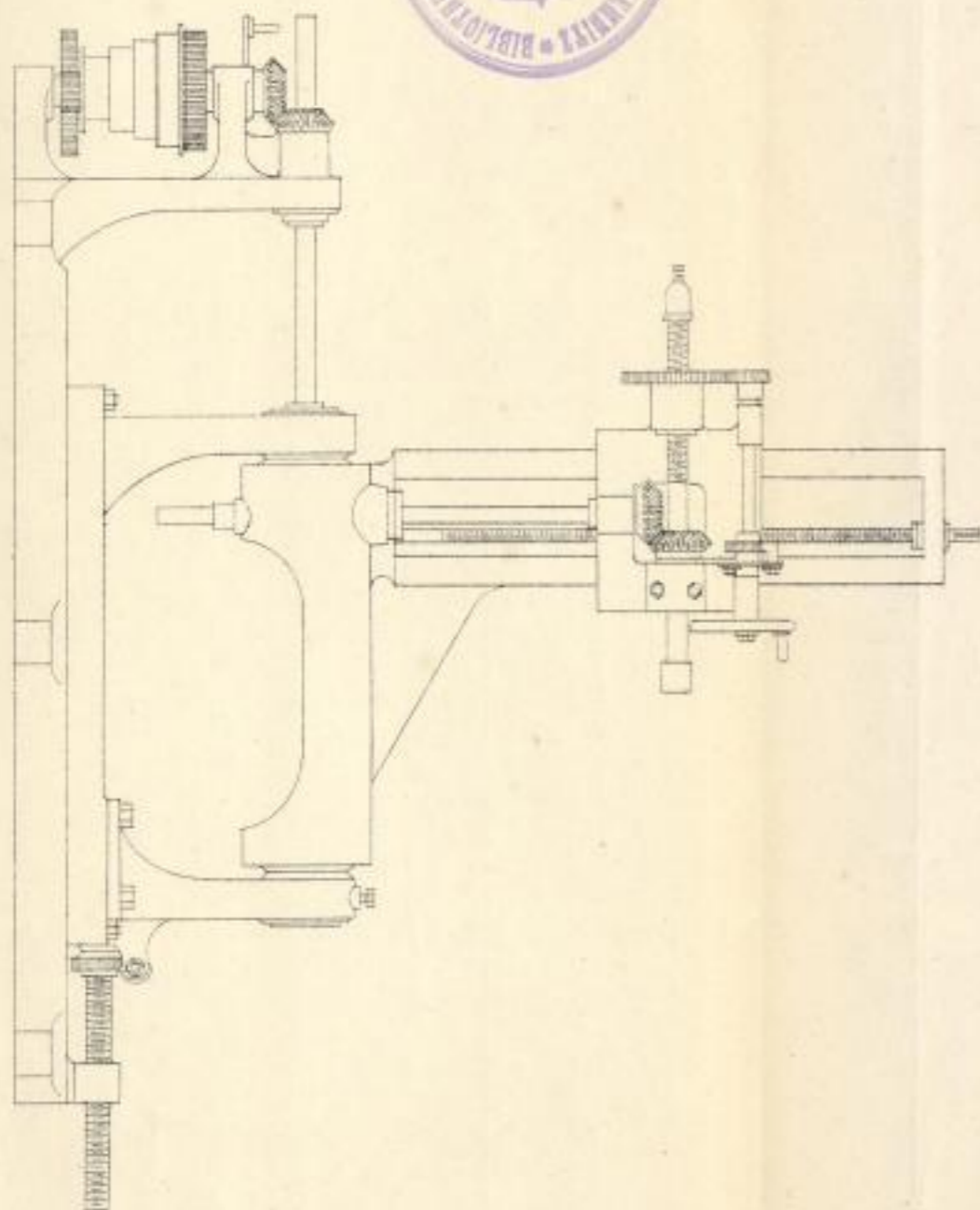
Wandradialbohrmaschine von Collet & Engelhard
