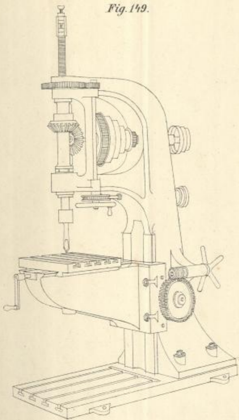
Freistehende Bohrmaschine der Werkzeugmaschinenfabrik Saxonia
