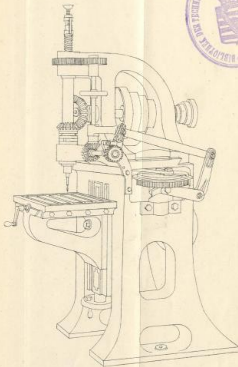
Freistehende Bohrmaschine der Werkzeugmaschinenfabrik Saxonia
