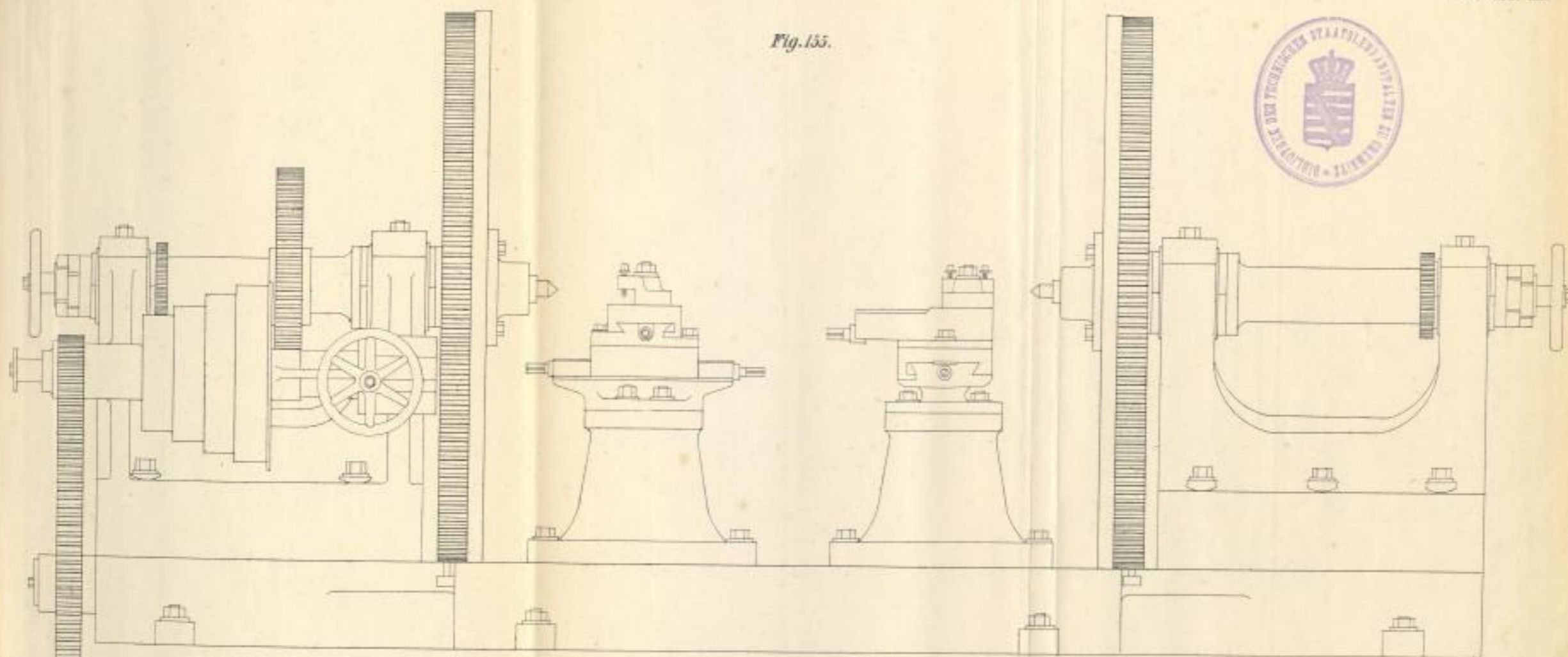
Räderschleifbank der Ottakringer Eisengiesserei und Maschinenfabrik.
