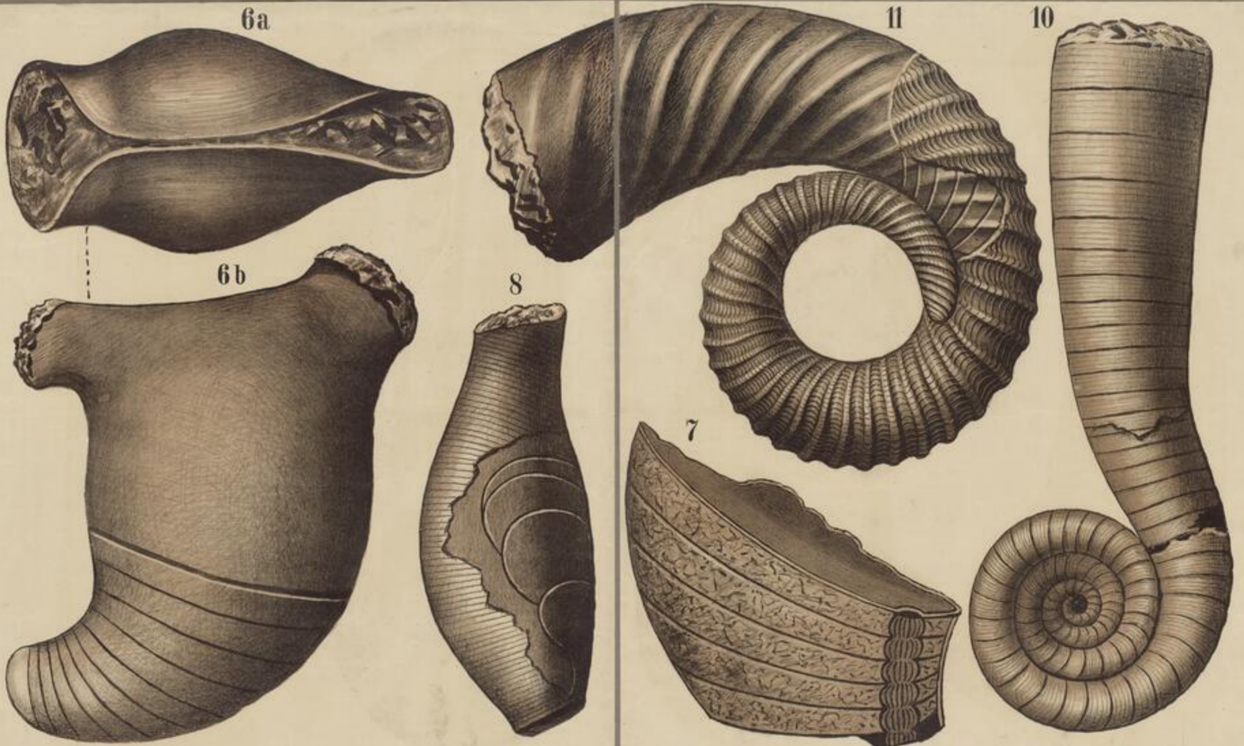
1. Orthoceras timidum. 2. O. Michelini. 3. Endoceras duplex 4. Cyrtoceras corbulatum. 5. Gomphoceras Bohemicum. 6. Phragmoceras Broderipi. 7. Ph. Loveni. 8. Ascoceras Bohemicum. 9. Ophidoceras simplex. 10. Lituides lituus. 11. Trochoceras optatum.
