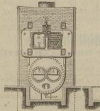
Dampfkessel nach bewährten Systemen.
