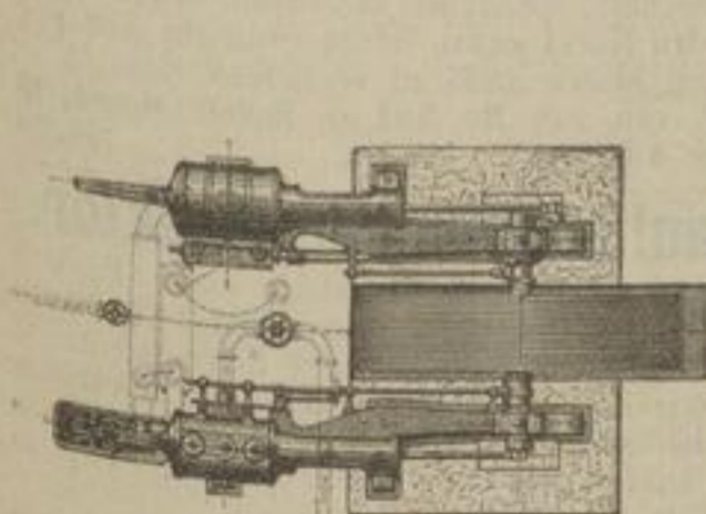
Dampfmaschinen mit Collmann-Steuerung.
