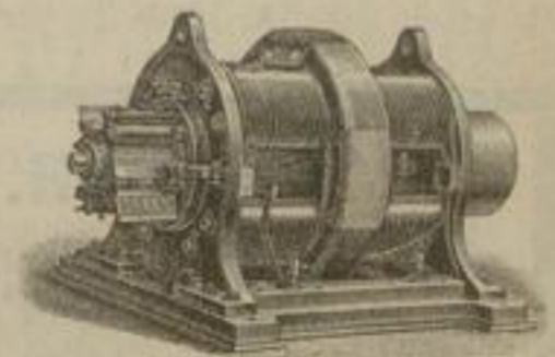
Elektrische Beleuchtung nach Patent Gülcher.
