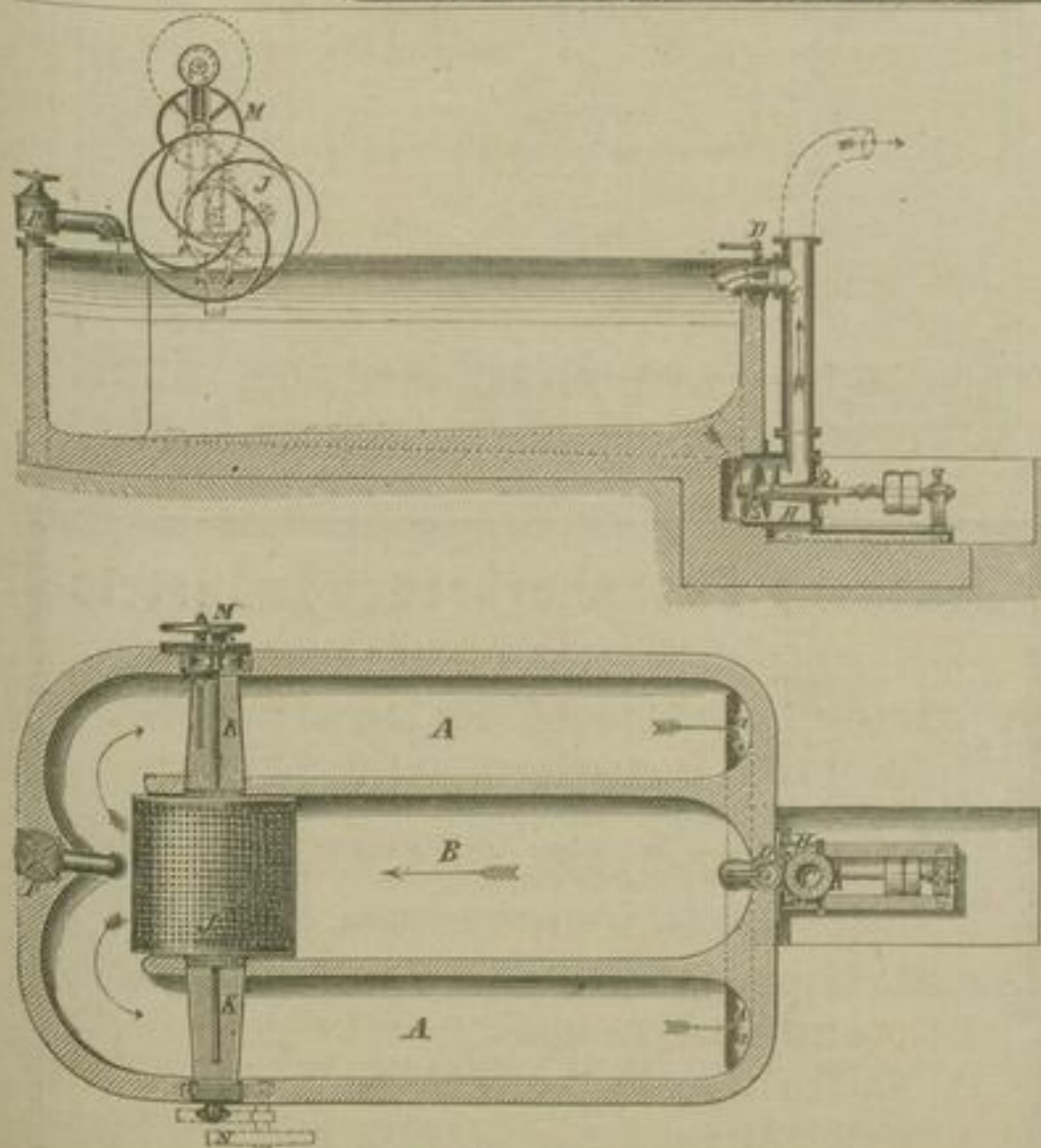
Celluloseauflös., Wasch- und Bleich-Holländer.
