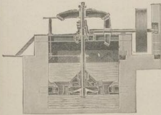
Niederdruck-Turbine an stehender Welle, 1-, 2- oder 3-kränzig.
