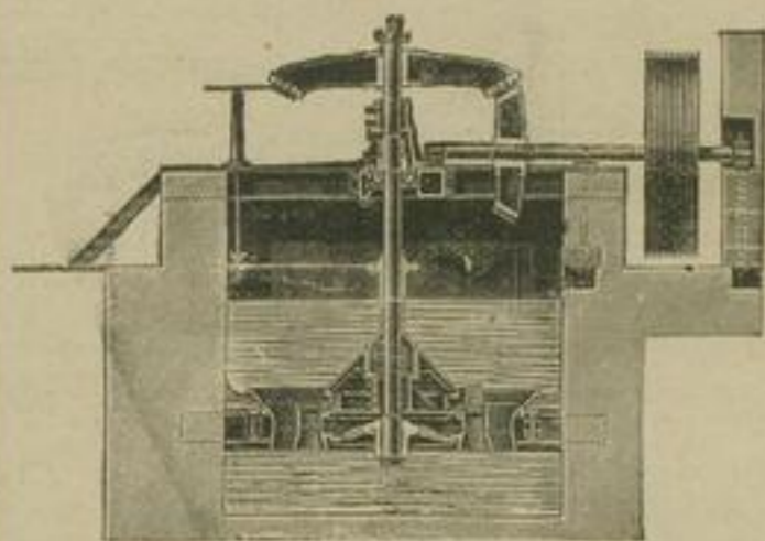
Niederdruck - Turbine an stehender Welle, 1-, 2- oder 3-körnig
