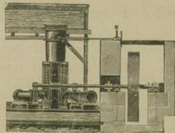
Hochdruck - Turbine an liegender Welle, 1- und 2-körnig; auf Wunsch auch mit hydraulischem Präcisionsregulator, z. B. für Elektricitätswerke etc.
