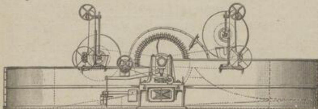
Halbzeugholländer, 500 kg Stoffeintragung.
