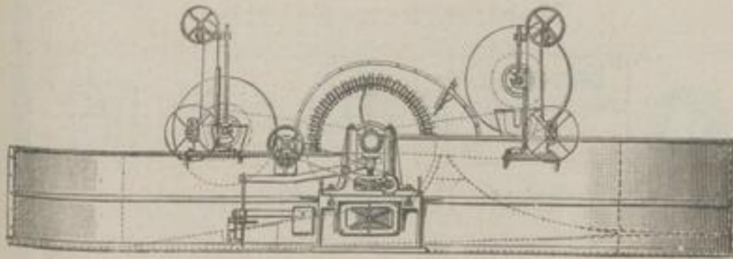
Halbzeugholländer, 500 kg Stoffeintragung.
