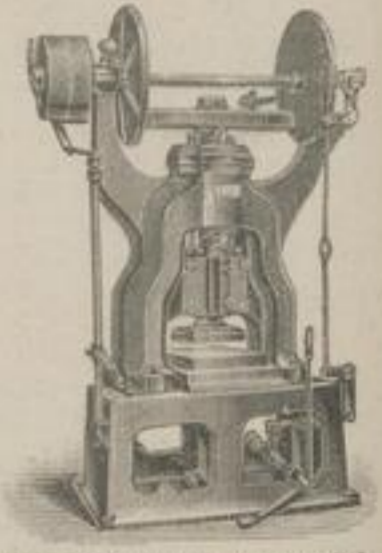
Balancier für Dampftrieb.
