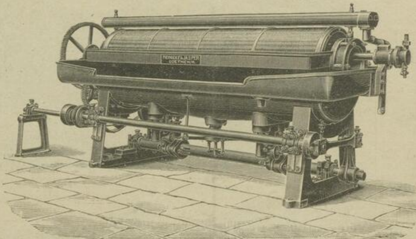
Rotirender Knotenfang mit lautloser Schüttlung. Pat. Reinicke & Jasper.
