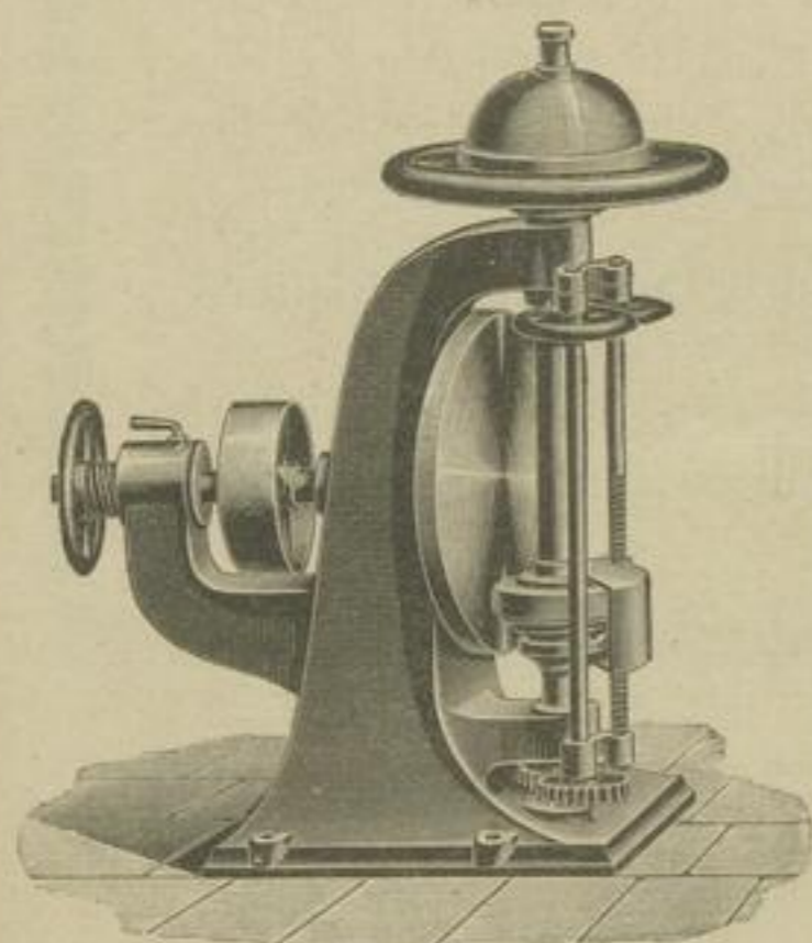
Schüttelbock für Papiermaschinen, Geschwindigkeit u. Hub während des Ganges verstellbar. Patent angemeldet.
