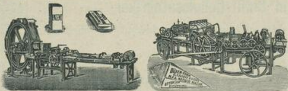
Papiersackmaschine.
