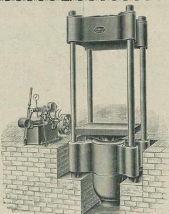
Hydraulische Presse.
