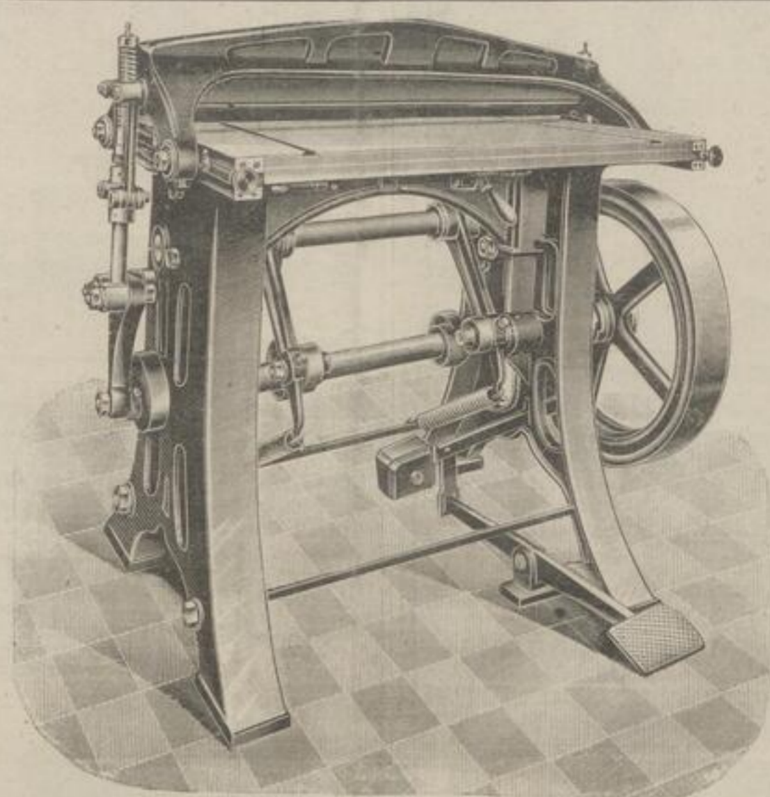
Pappenstauchmaschine für Dampftrieb mit 50, 75 und 100 cm Durchgangsraum.
