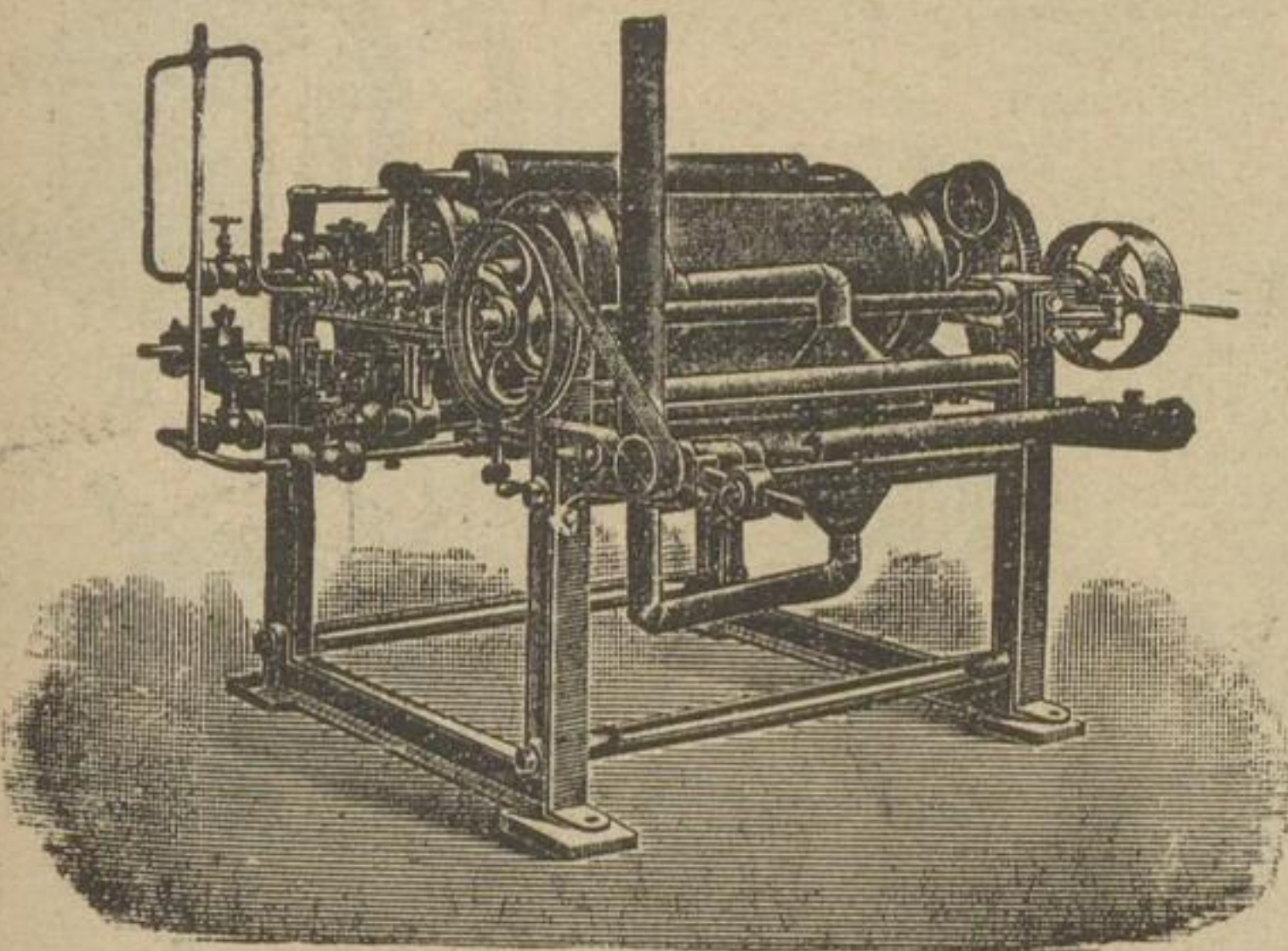
Maschine zur Herstellung von Paraffin- und Wachs-Papier
