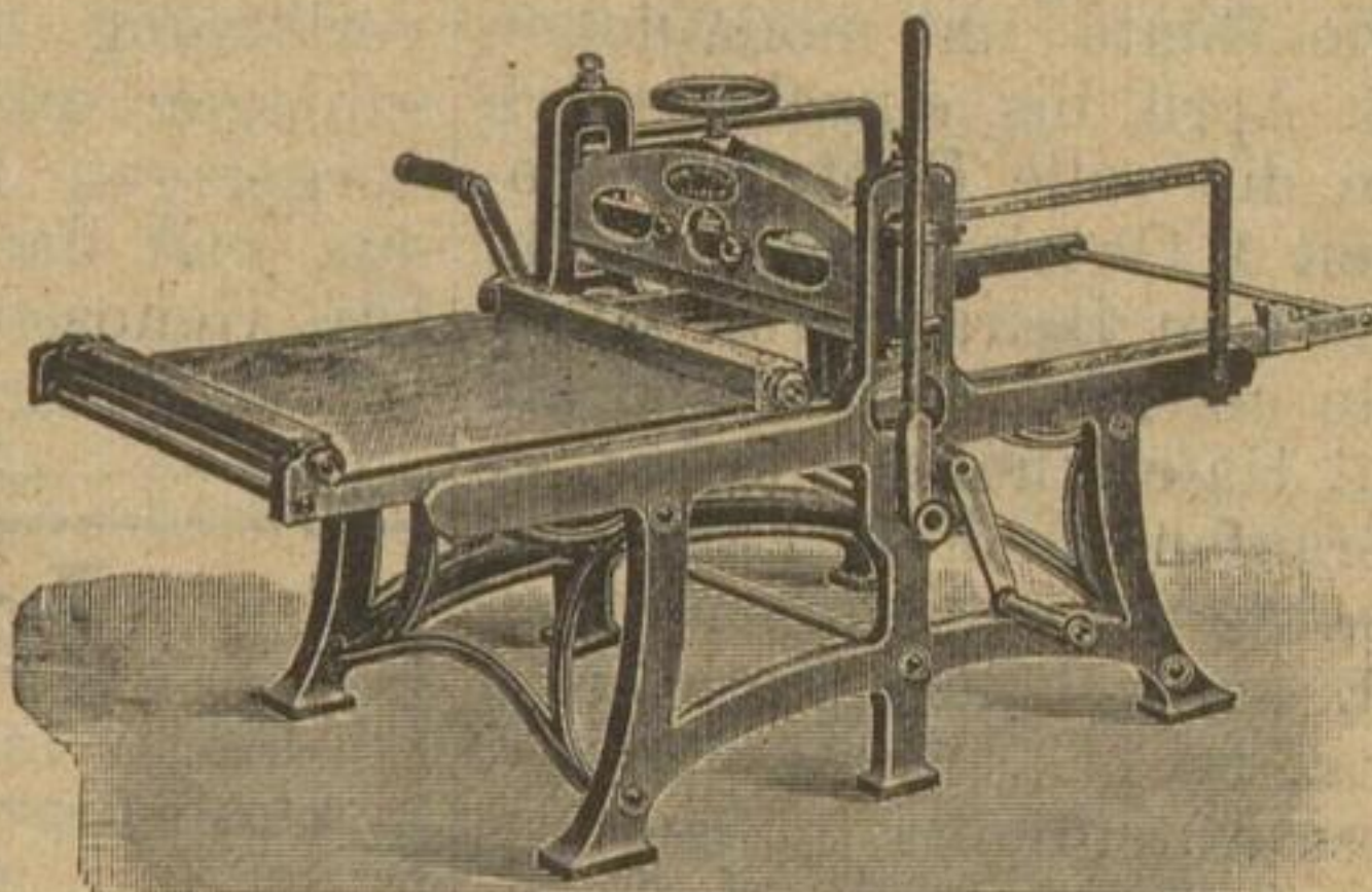
Leichte Steindruckhandpresse SHL
