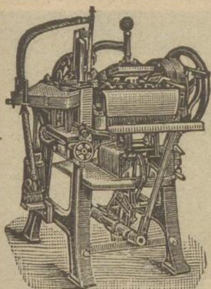
Briefumschlagmaschine mit einfacher Gummirung
