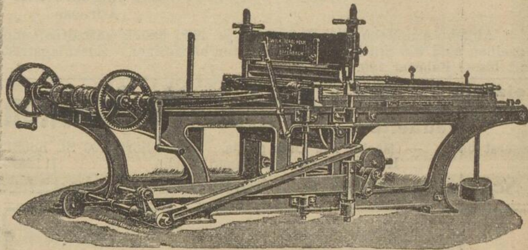
Tritthebelpresse
