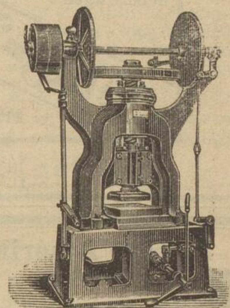
Balancier für Dampfbetrieb
