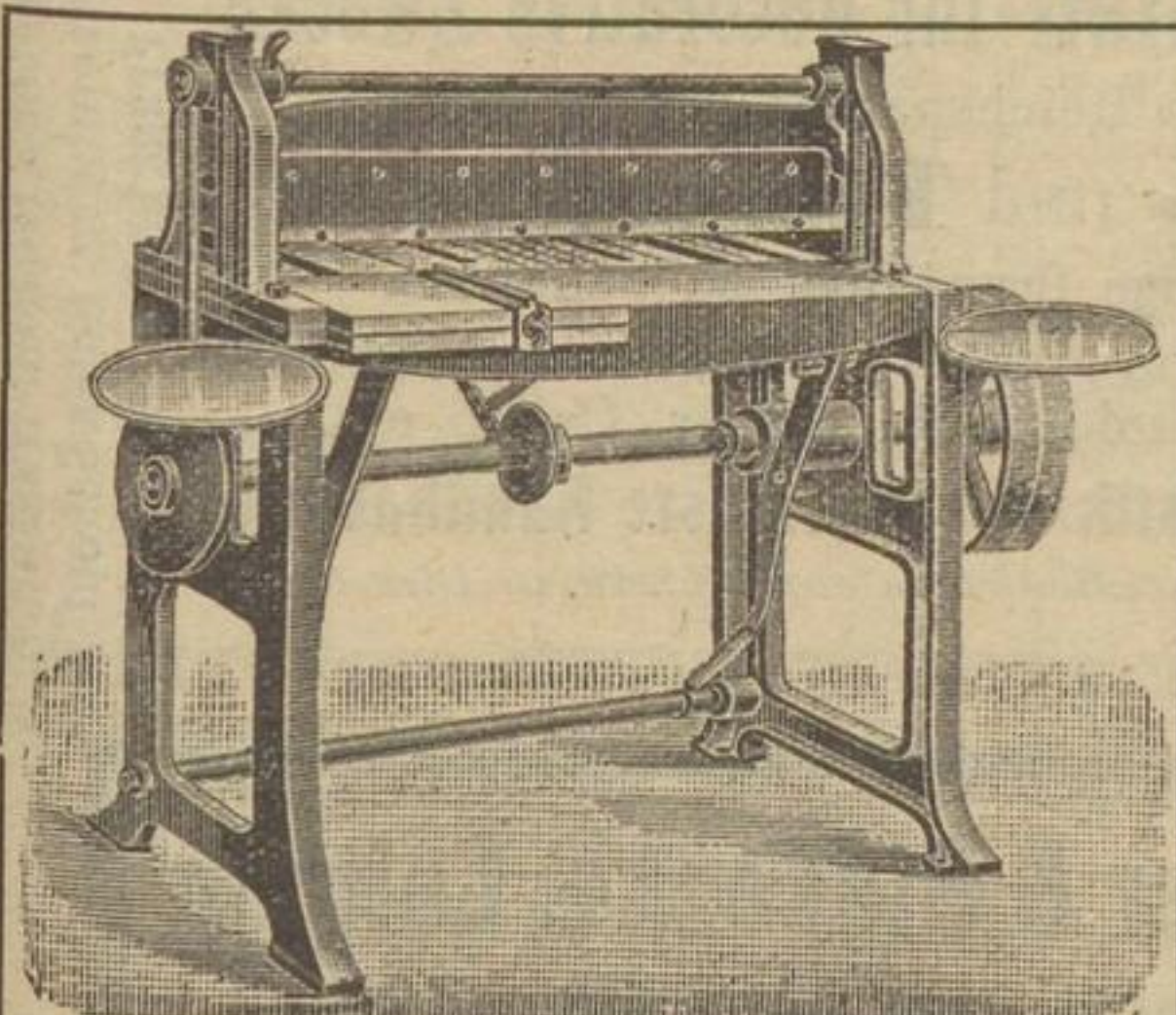
Universal-Pappenbiegemaschine „No. 35“ DRP biegt selbst die sprödesten Pappen tadellos, und arbeitet gleichzeitig mit beliebiger Anzahl verstellb. Messer. „Ersetzt 3 Maschinen.“ Bietet also grosse Ersparnisse.
