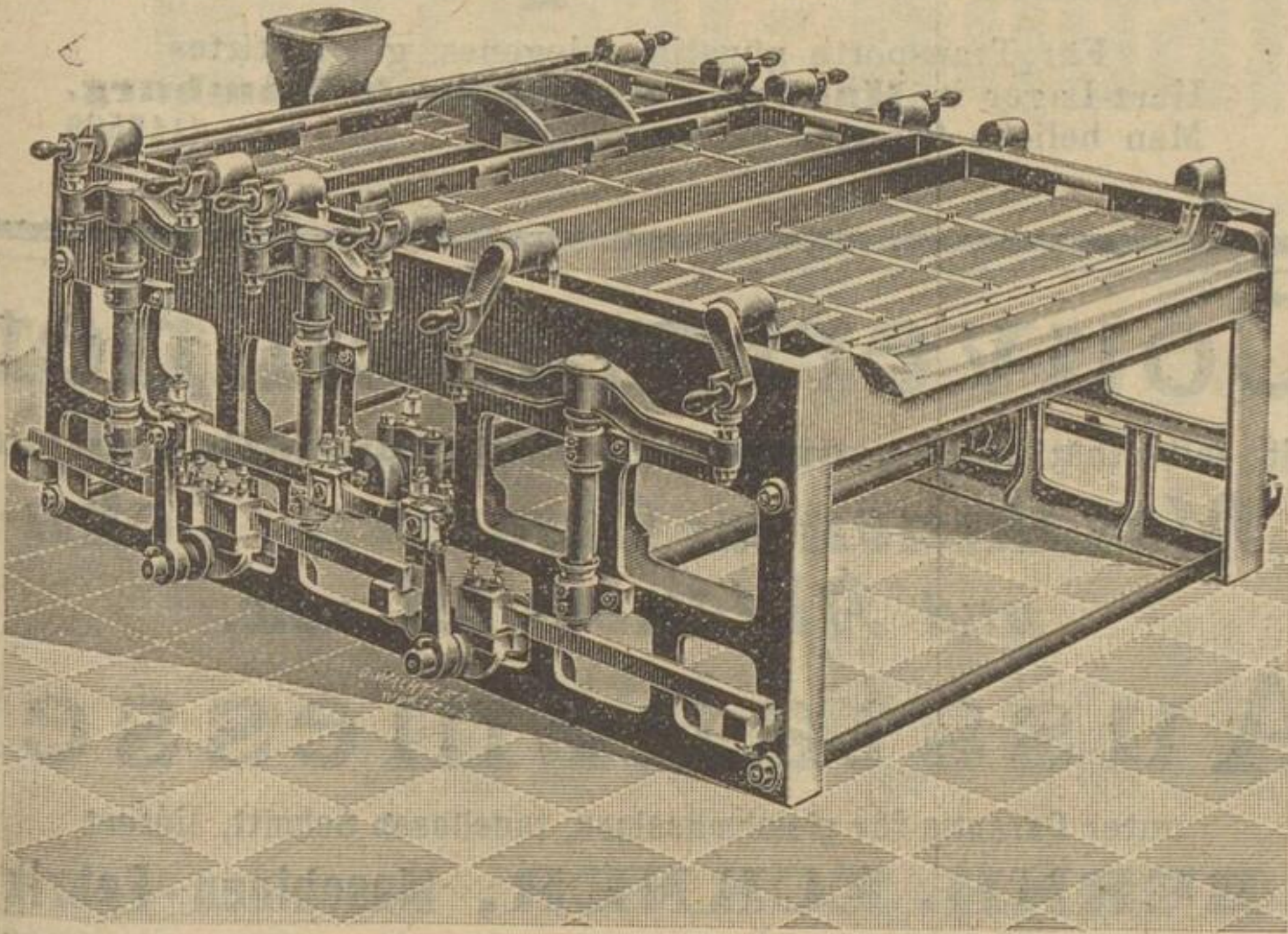
Plan-Knotenfang mit 3 Platten-Behältern in einem Stoffbehälter geräuschlose Central-Schüttlung.
