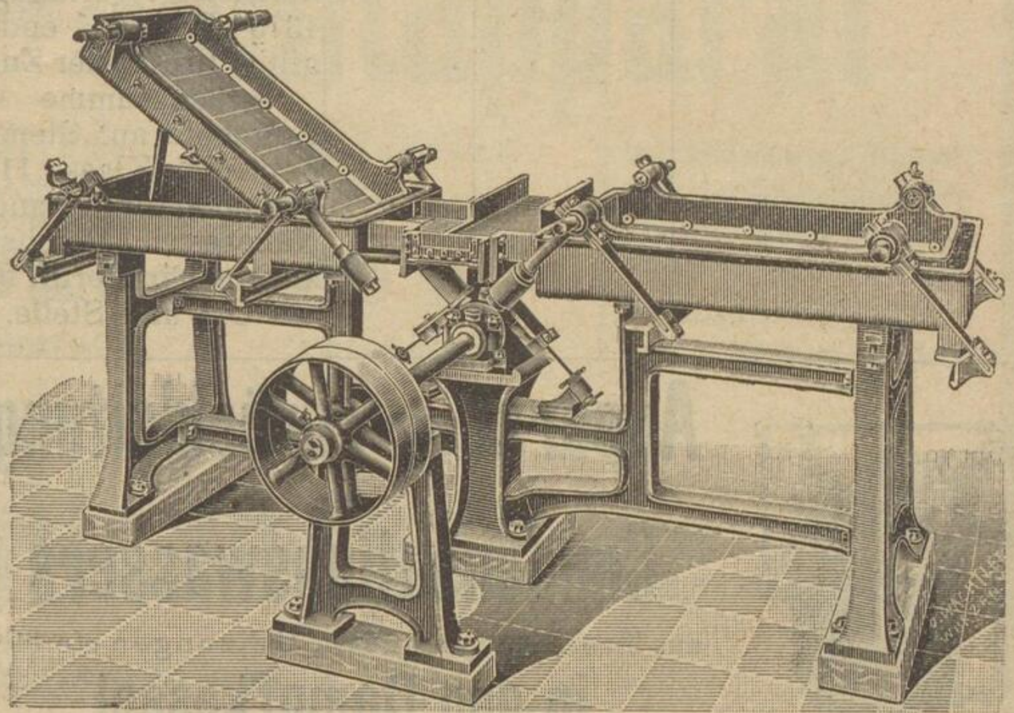
Planknotenfang mit Diagonal-Schüttlung D. R.-Pat. No. 87963 (Schmidt & Seybold).
