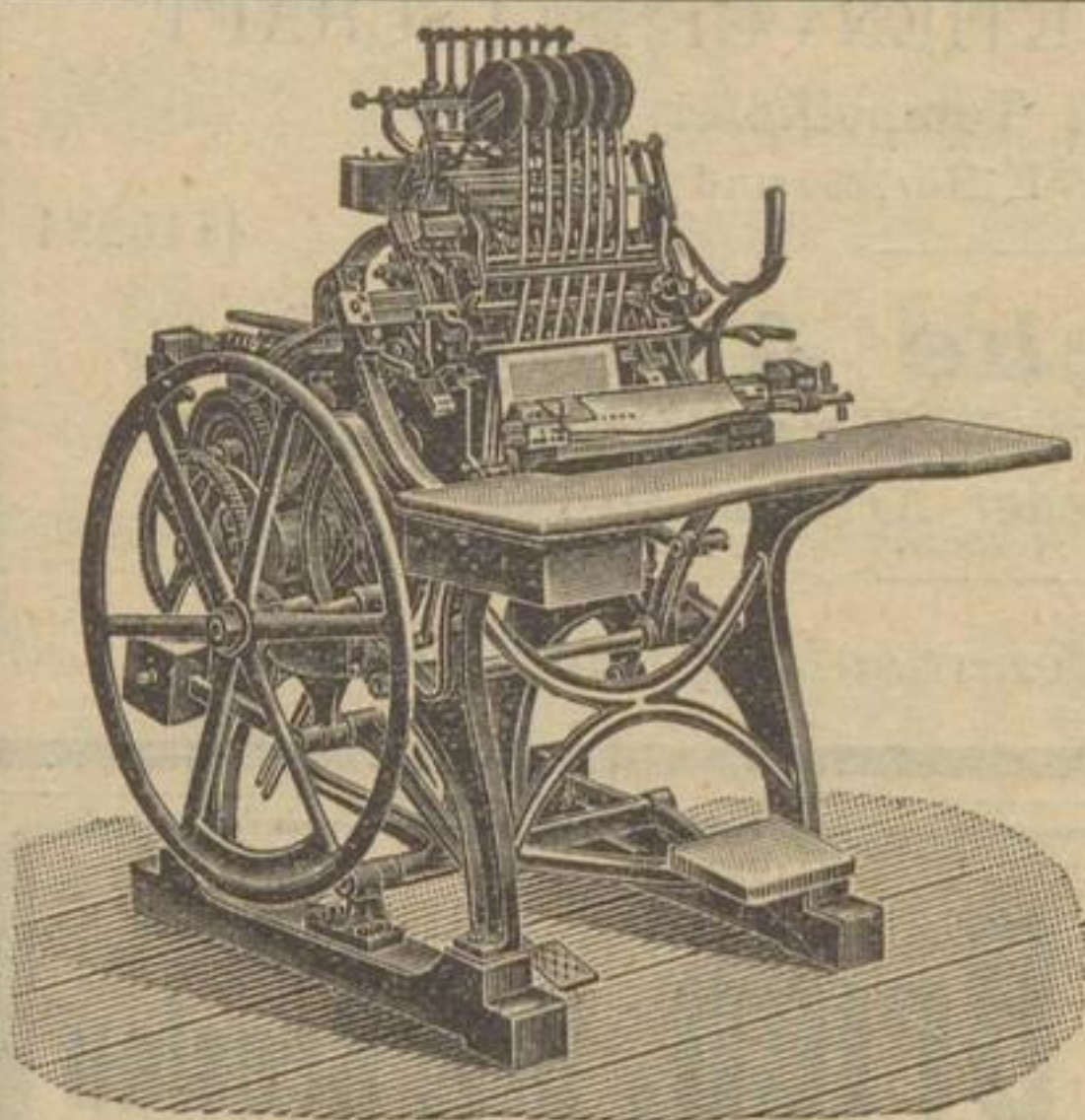
Faden-Heftmaschine No. 38 für Kraft- und Fussbetrieb
