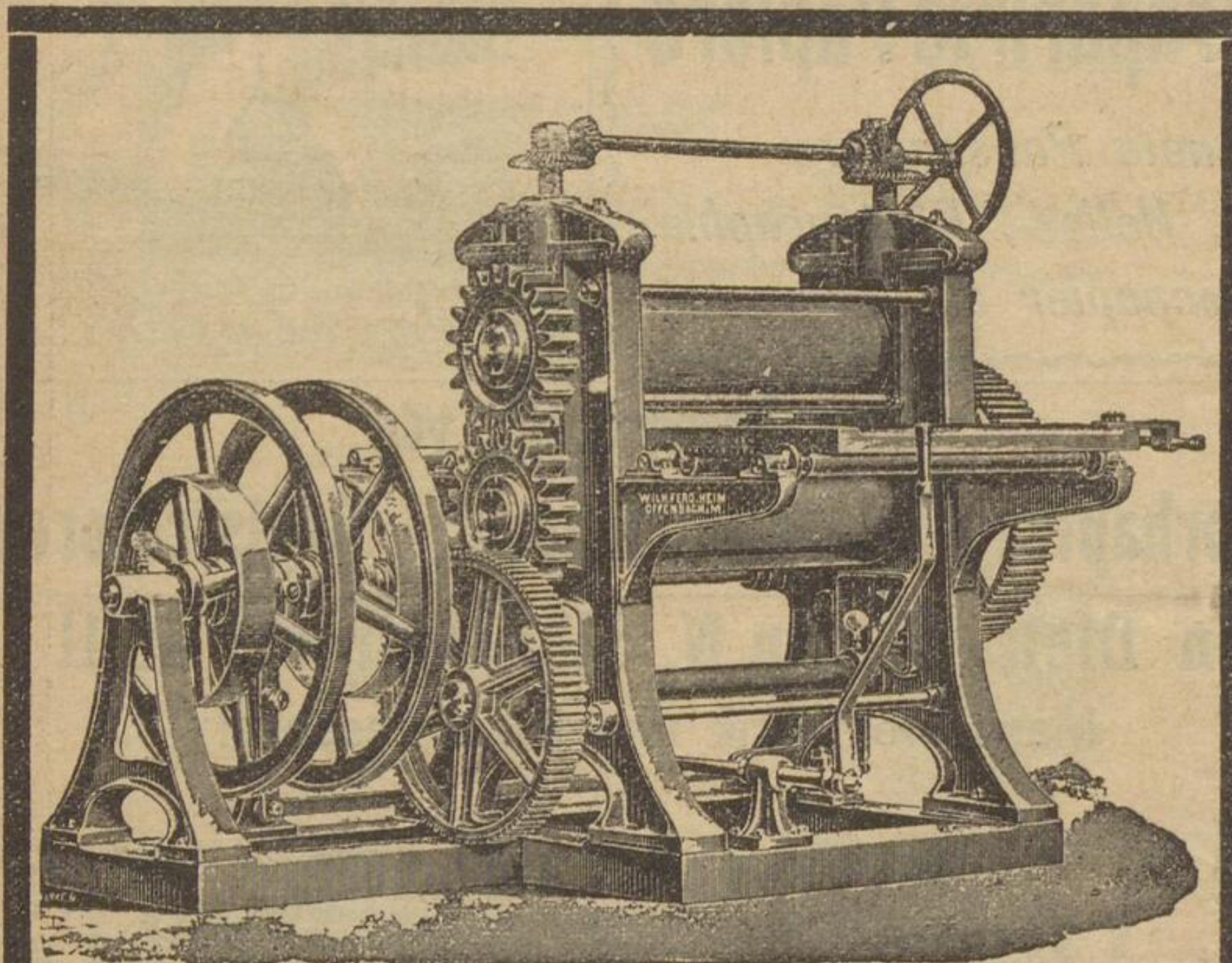
Schweres Walzwerk zum Prägen und Ausschneiden
