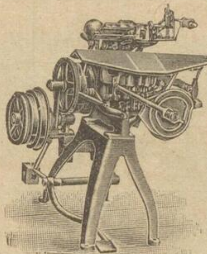
Faden-Heftmaschine für Schreib- u. Zeichen-Hefte mit selbstth. Verknotung des Fadens.
