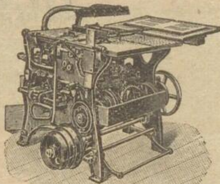
Octav-Falzmaschine für 3 Bruch mit Faden-Heftapparat zum gleichzeitigen Holländern der gefalzten Bogen.
