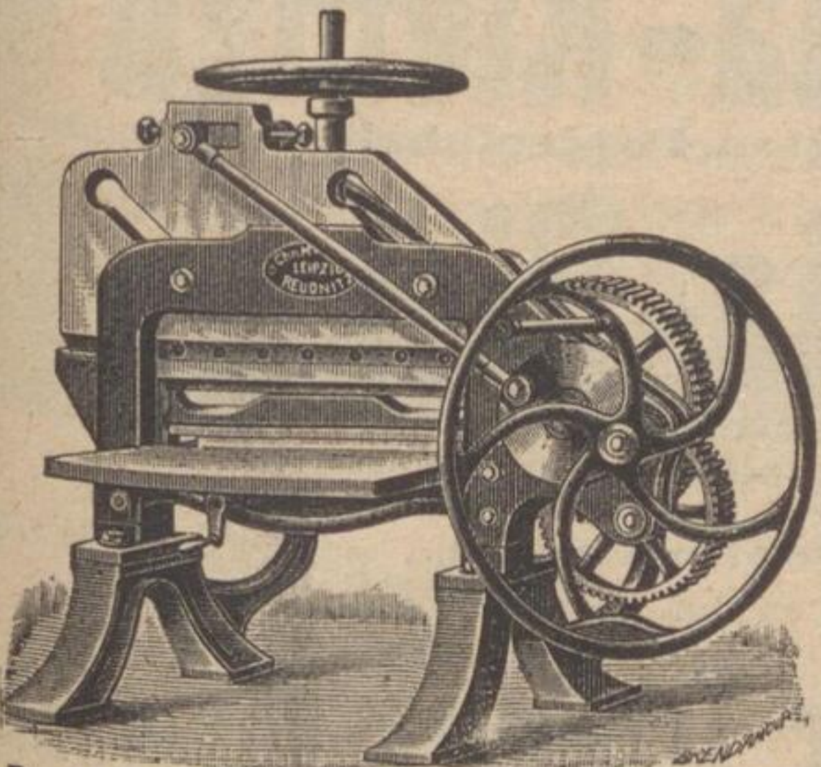
Papier-Schneidemaschine (Radsystem) mit verbesserter Handpressvorrichtung.
