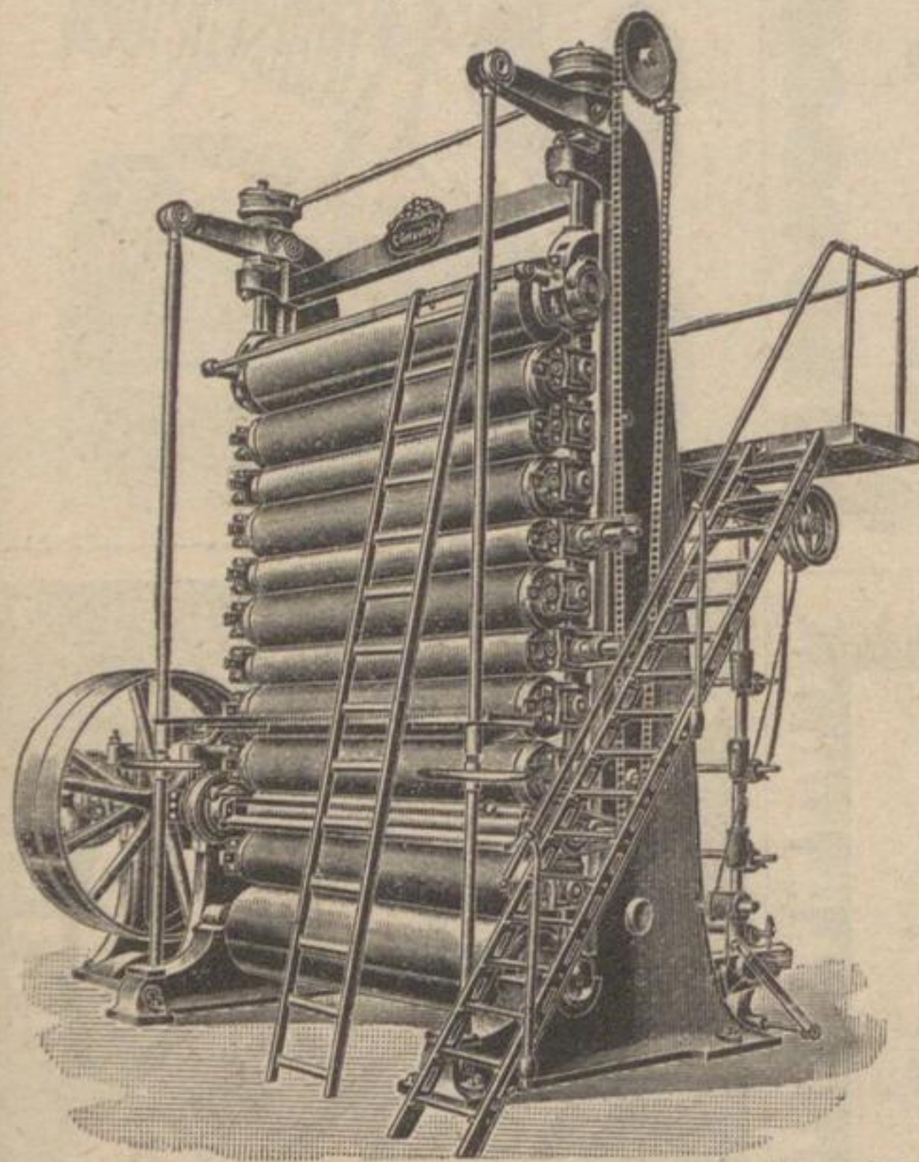
Rollen-Calander mit 12 Walzen und directem Antrieb der 3. Walze f. 2 Geschw. u. 1 Riemen.
