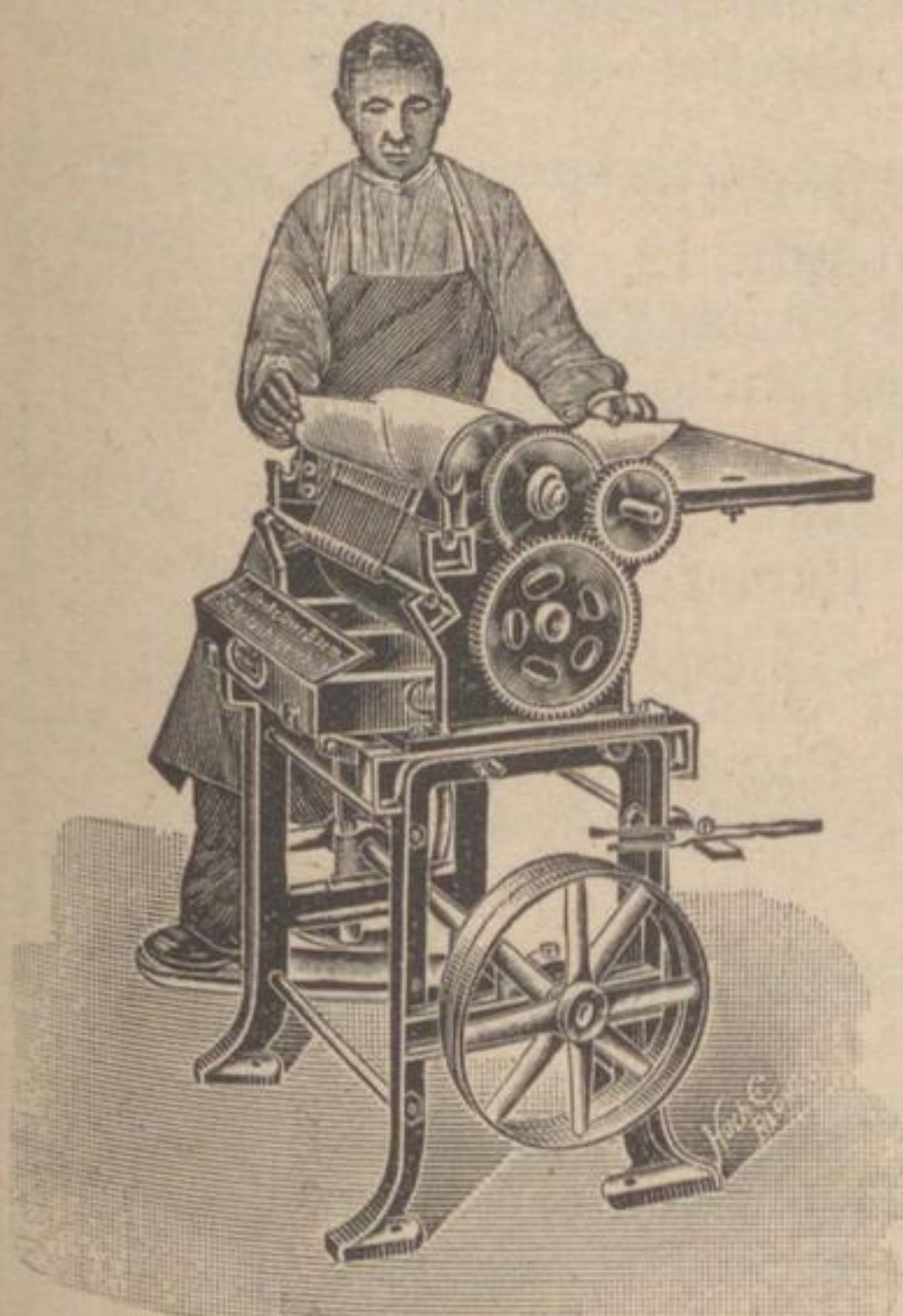
Bogen-Anleimmaschine Mod. B
